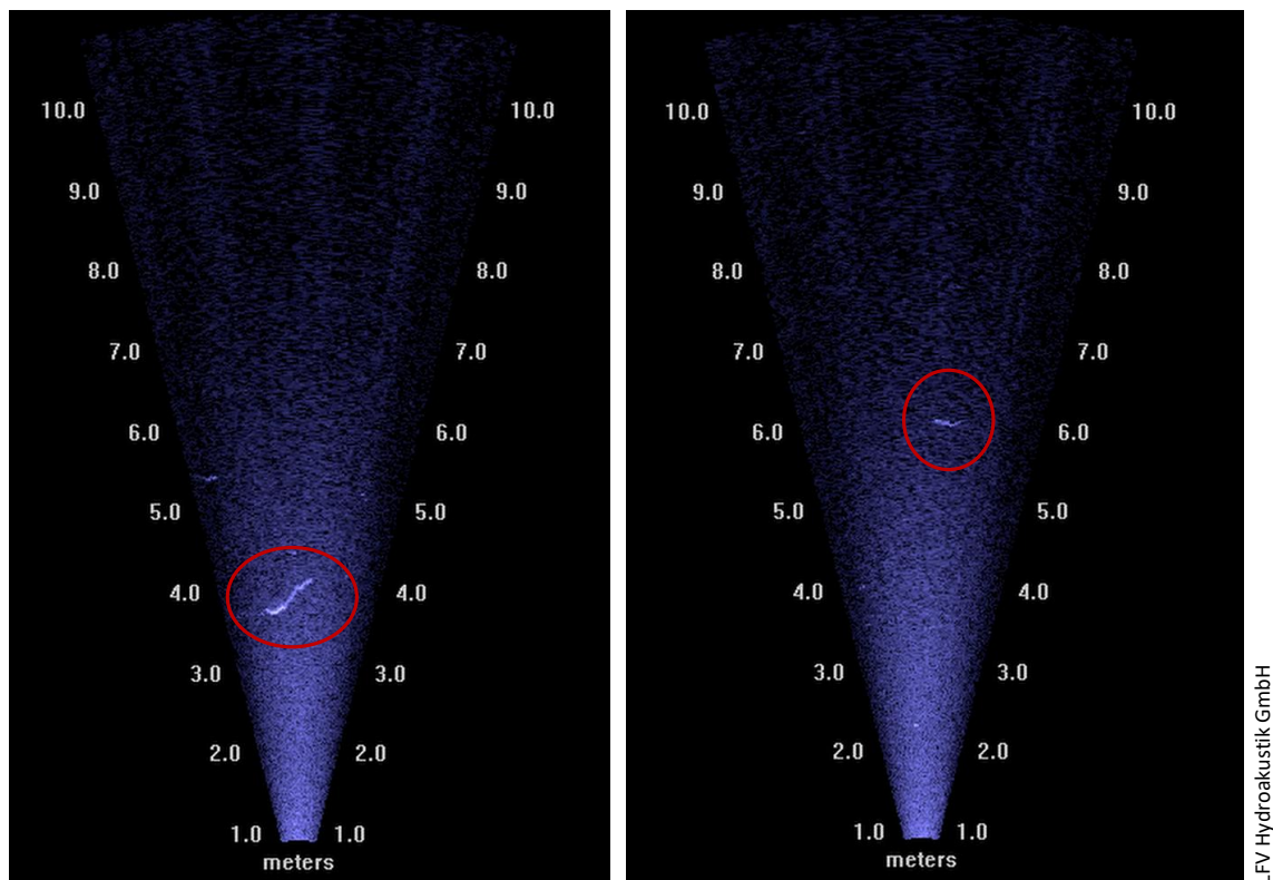
Abb. 51: Ausschnitte aus DIDSON-Sequenzen: links ein absteigender Aal, rechts ein aufsteigendes Neunauge. Der Schallkegel richtet sich vom rechten Ufer in Richtung Gewässermittle, so dass die Fließrichtung in den Ausschnitten von links nach rechts ist. Die Zahlen geben den Abstand [m] zum Sonarkopf an.
