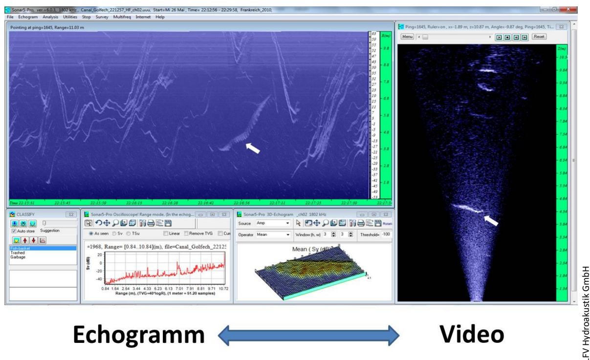
Abb. 50: Beispielhafter Screenshot aus Sonar 5 Pro. Darstellung als Echogramm (links) mit korrespondierendem Video (rechts). Weißer Pfeil markiert links eine Fisch-Spur „trace“ und rechts das zugehörige Fischecho im Video.
