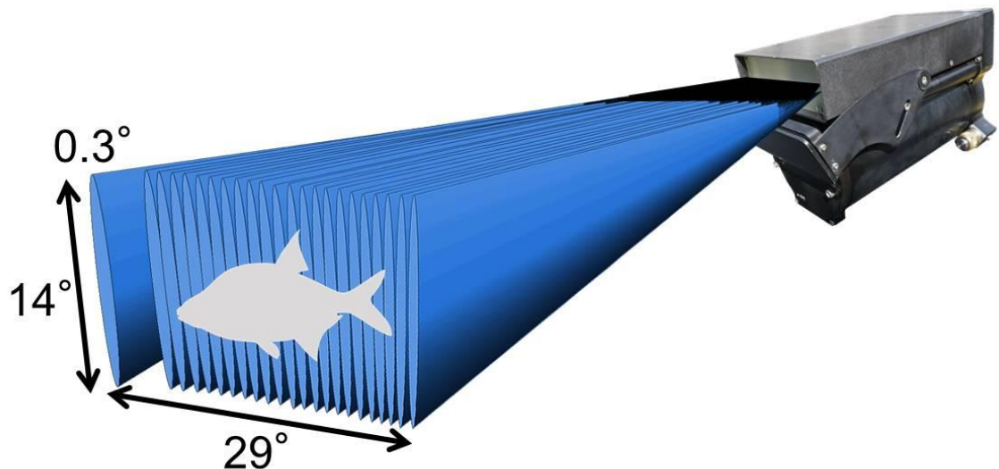
Abb. 49: Schematische Darstellung des DIDSON Schallkegels
