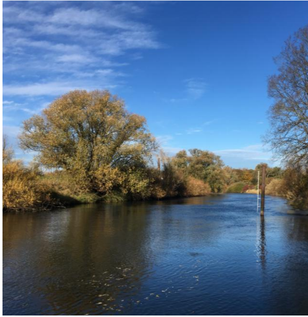
Abb. 47: Standort des Sonars in der Lippe bei Wesel (km 3) (links, Blickrichtung flussabwärts), das DIDSON wurde mit einer speziell dafür angefertigten Halterung an einem alten Pegel befestigt (rechts).
